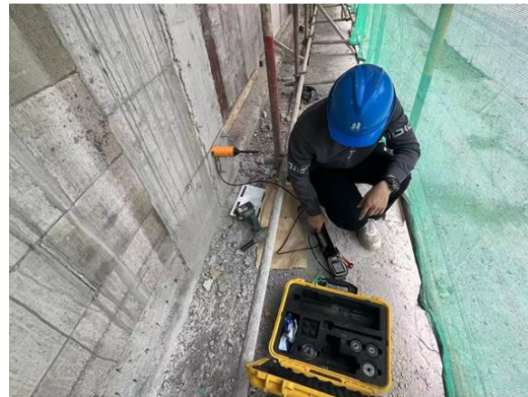
(后置埋件拉拔试验)
