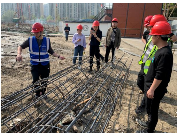
(钢筋笼现场抽查)
