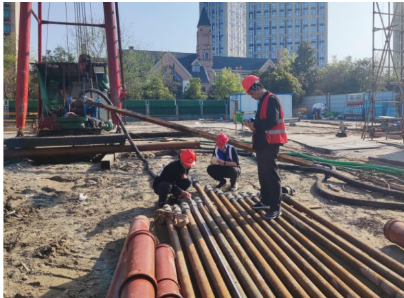
(桩基钻杆长度检查)
